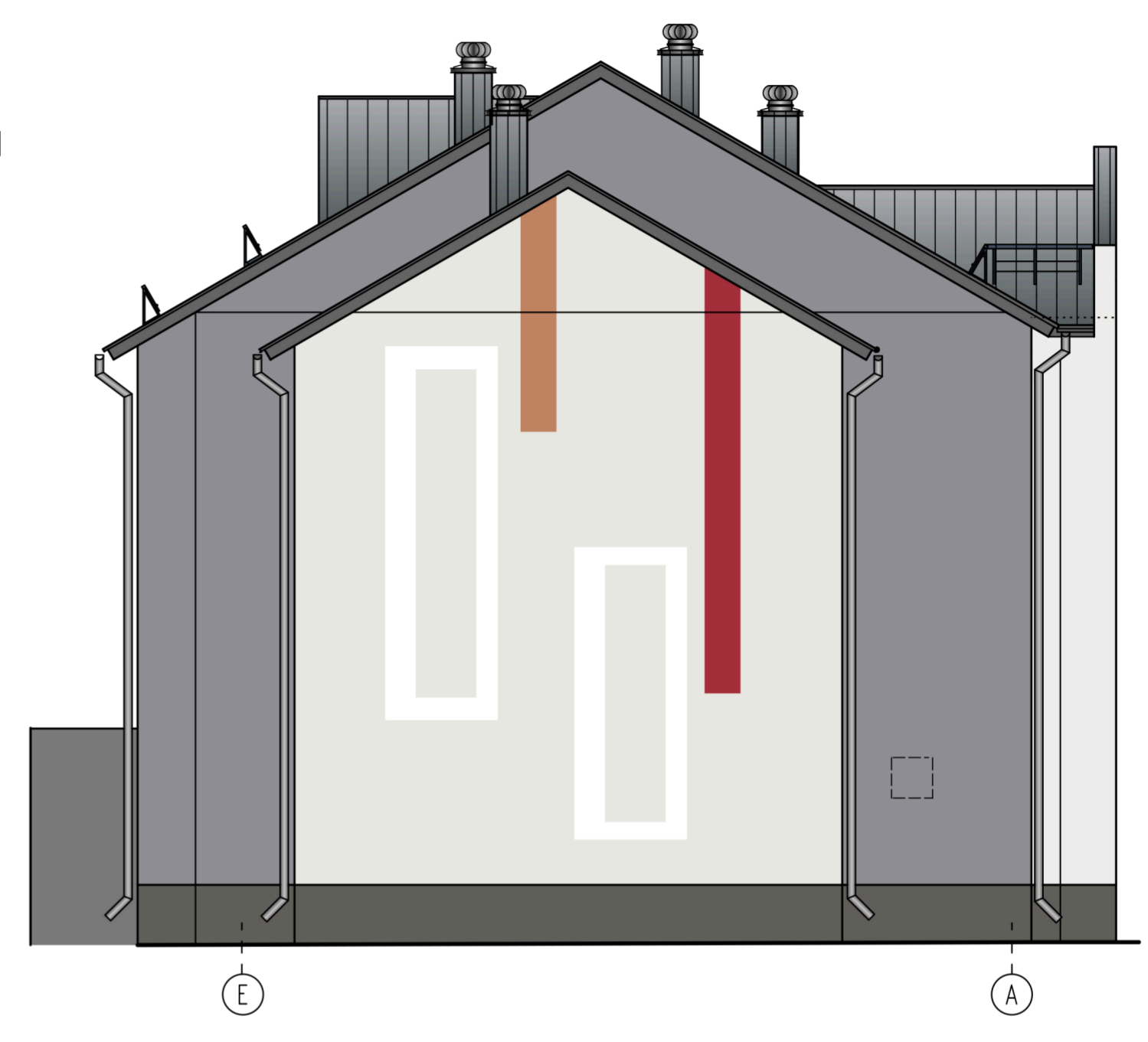
ФАСАД Е-А
